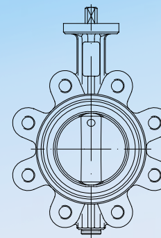
▶ 015 – DN 80 lug type butterfly valve
