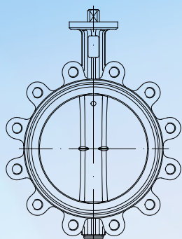
▶ 015 – DN 200 lug type butterfly valve
