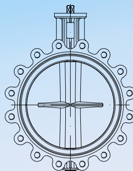
▶ 015 – DN 350 lug type butterfly valve
