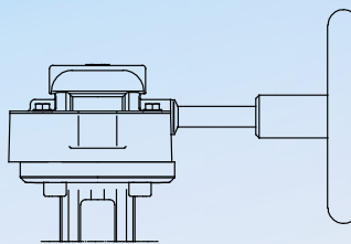
► 014/015 – with worm gear
